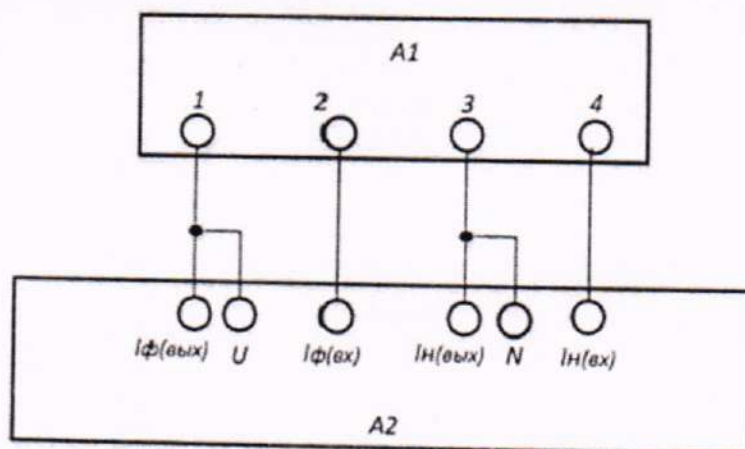
Рисунок 2 – Схема подключения однофазного счетчика к поверочной установке
