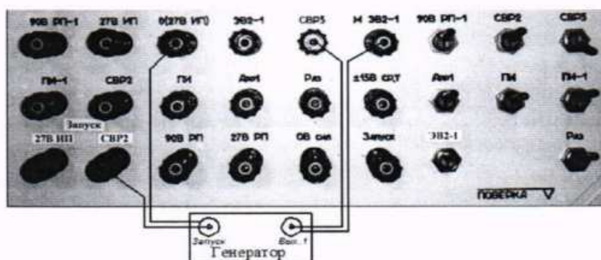
Рисунок 42 – Схема измерения системой времени воспроизведения команды «СВР5»
