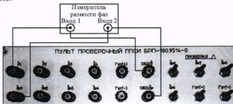
Рисунок 55 – Схема измерений разности фаз
