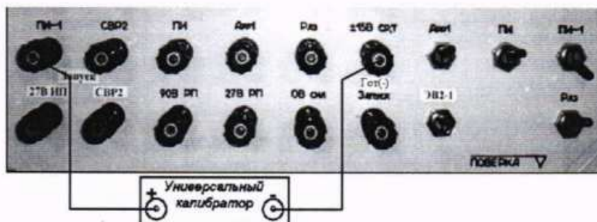
Рисунок 47 – Схема проверки напряжения постоянного тока команды «ПИ-1»
