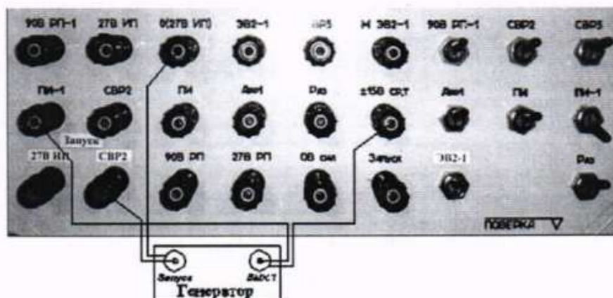
Рисунок 38 – Схема измерения системой времени задержки сигнала «ПИ-1»
