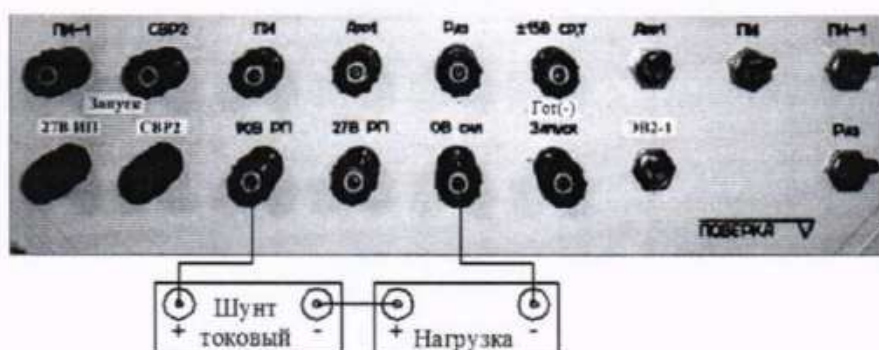
Рисунок 57 – Схема проверки при измерениях системой силы постоянного тока
