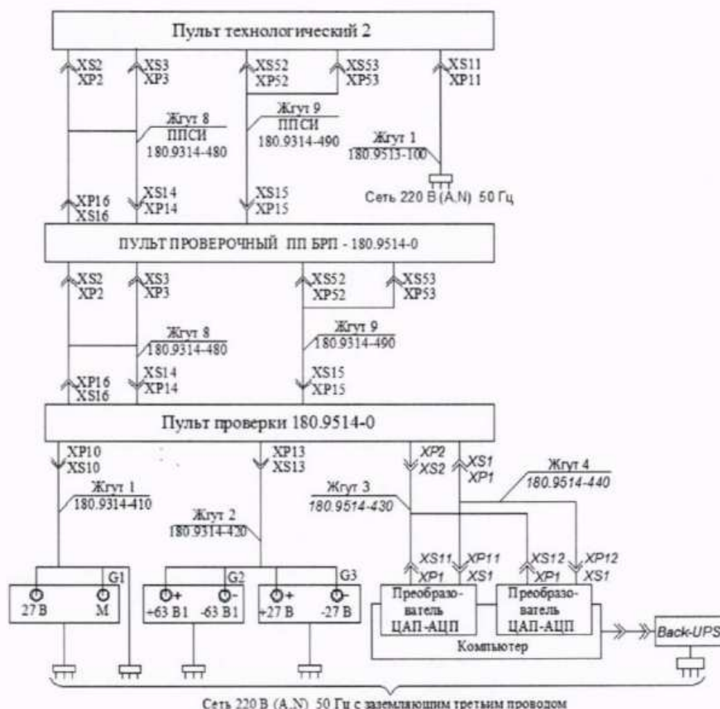
Рисунок 1 - Рабочее место для проверки системы № 012081 в автоматизированном режиме
