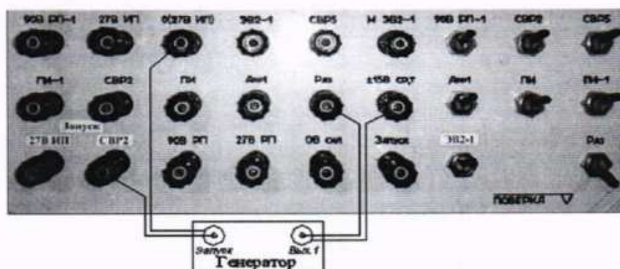
Рисунок 40 – Схема измерения системой времени задержки сигнала «Разар.»
