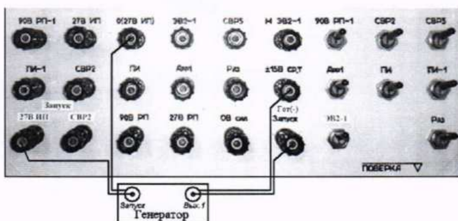
Рисунок 36 – Схема измерения системой времени задержки сигнала «Готов -»
