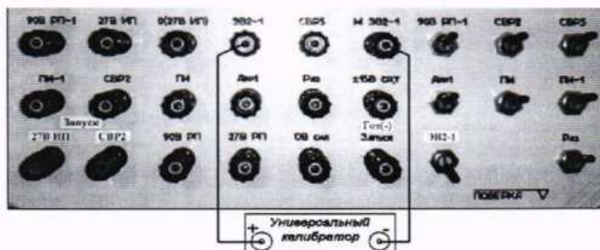
Рисунок 44 – Схема проверки напряжения постоянного тока команды «ПИ» по цепи «ЭВ2-1»
