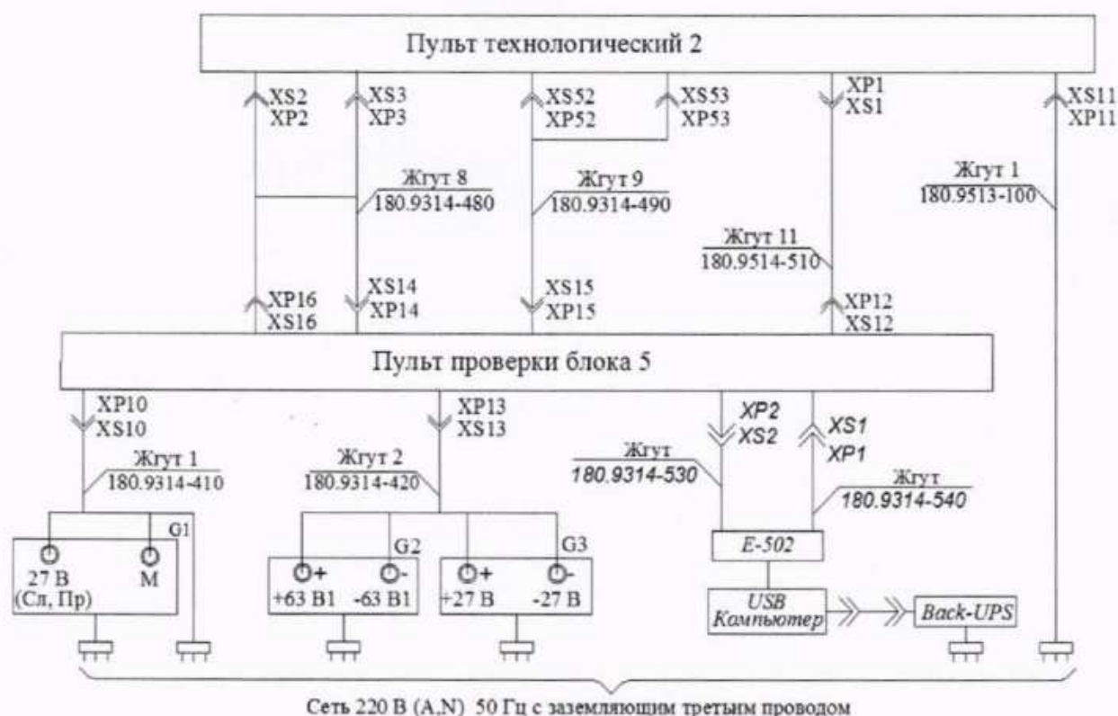
Рисунок 2 - Рабочее место для проверки системы № 202194 в автоматизированном режиме
