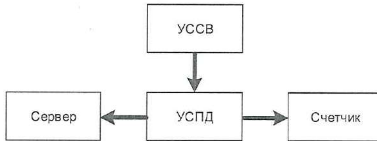
Рис. 2 – Логический канал передачи национальной шкалы времени UTC(SU) от резервного источника точного времени к компонентам СОЕВ
