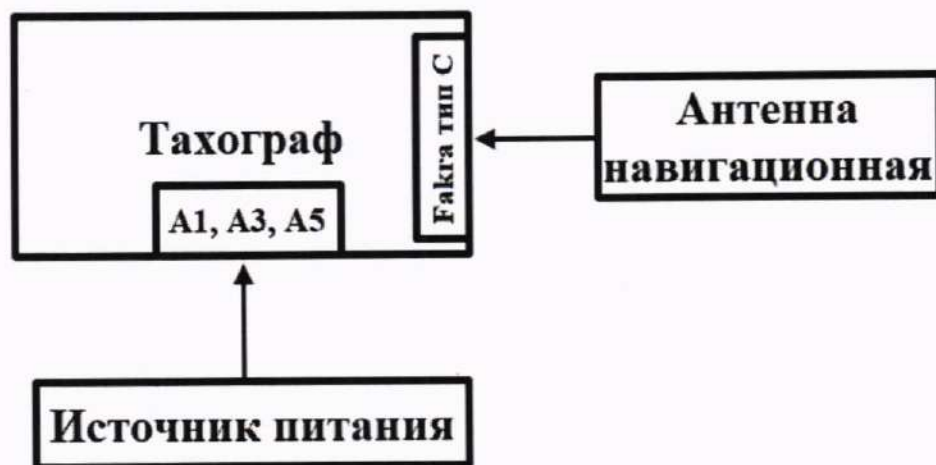
Рисунок 1 – Схема проведения измерений при опробовании
