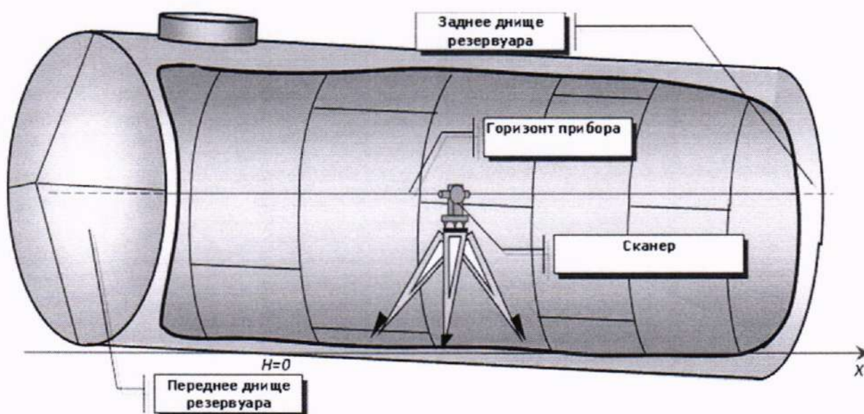
Рисунок 1 - Расположение сканера при измерениях внутри резервуара
