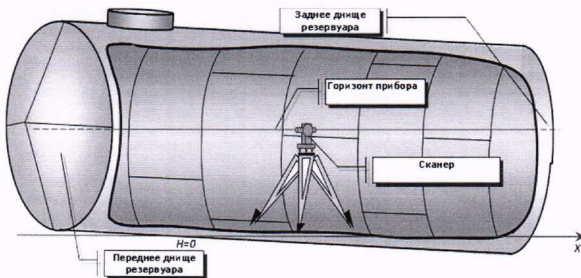
Рисунок 1 - Расположение сканера при измерениях внутри резервуара
