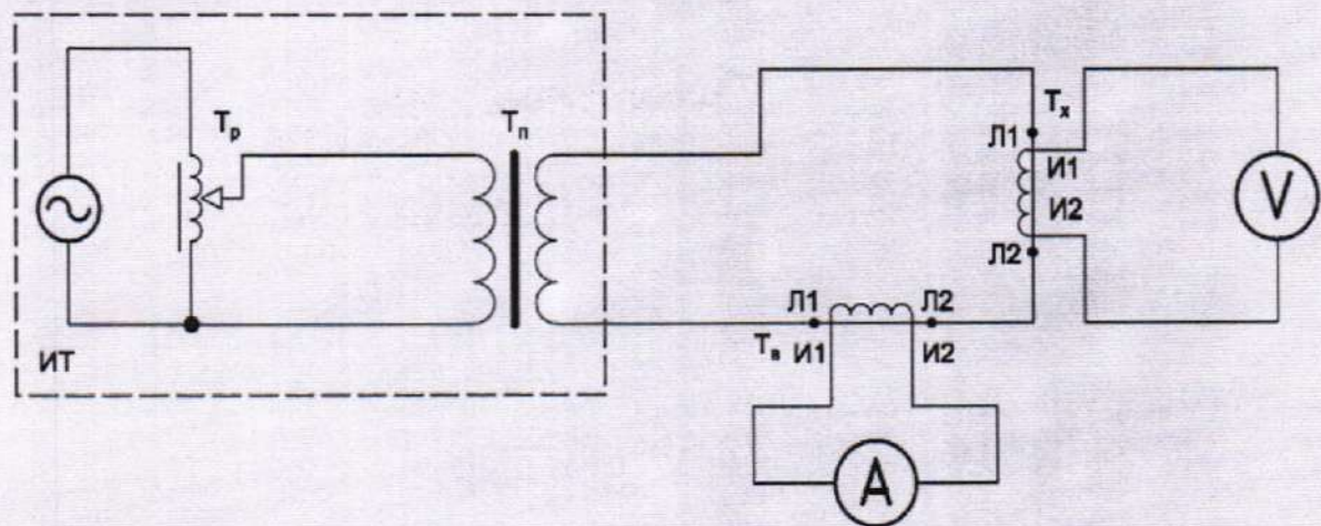
ИТ — регулируемый источник синусоидального тока; ~ — сеть (генератор); Т р — регулирующее устройство (автотрансформатор); Т п — понижающий силовой трансформатор; Т х — проверяемый трансформатор; Т а — вспомогательный трансформатор
