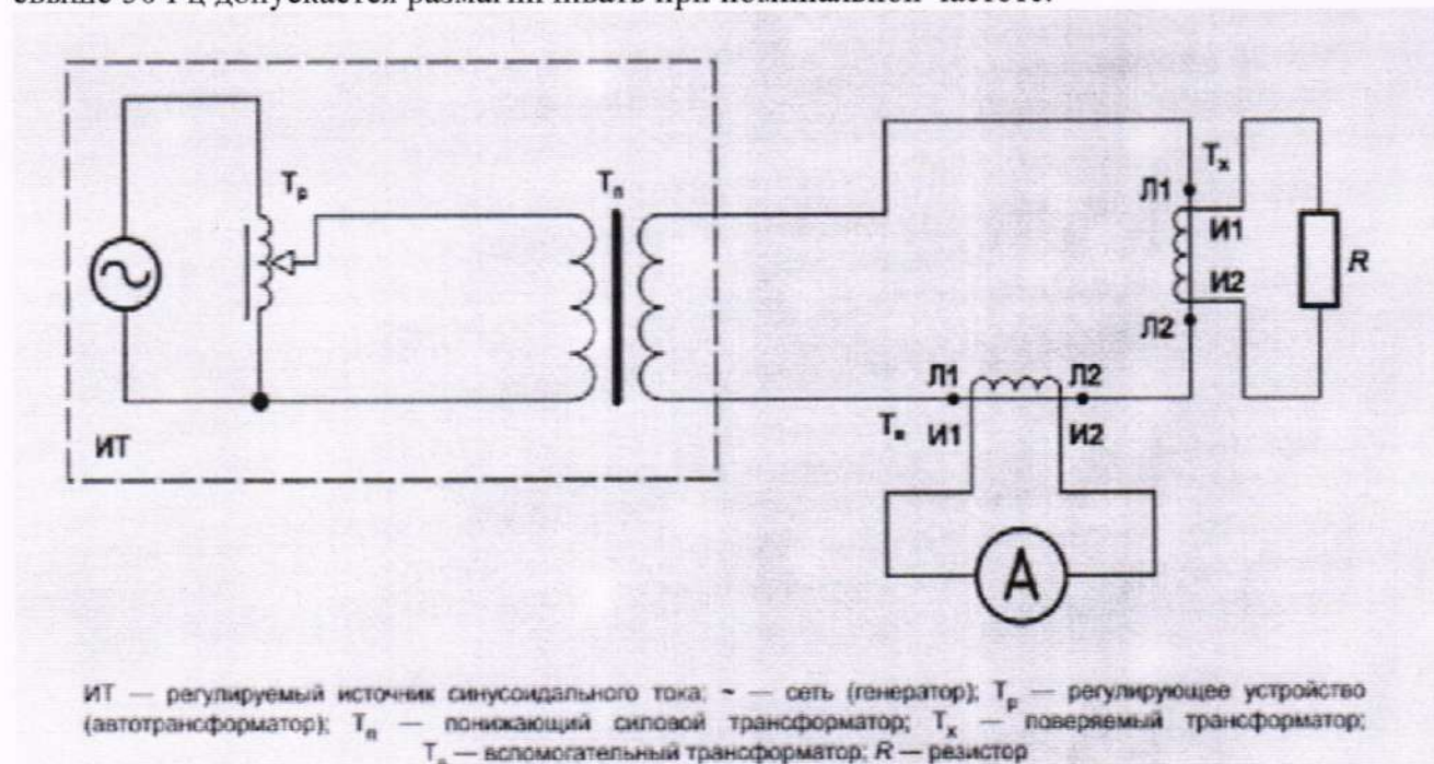
Рисунок 1 – Схема размагничивания трансформатора первым способом
