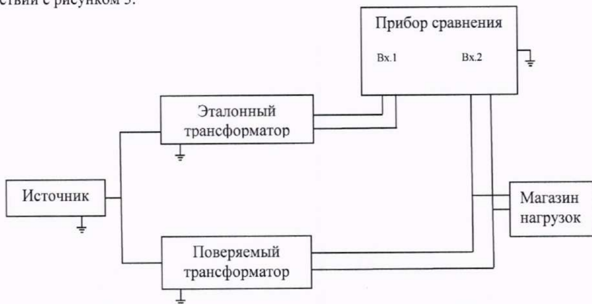
Рисунок 3 – Схема определения токовых и угловых погрешностей трансформаторов
