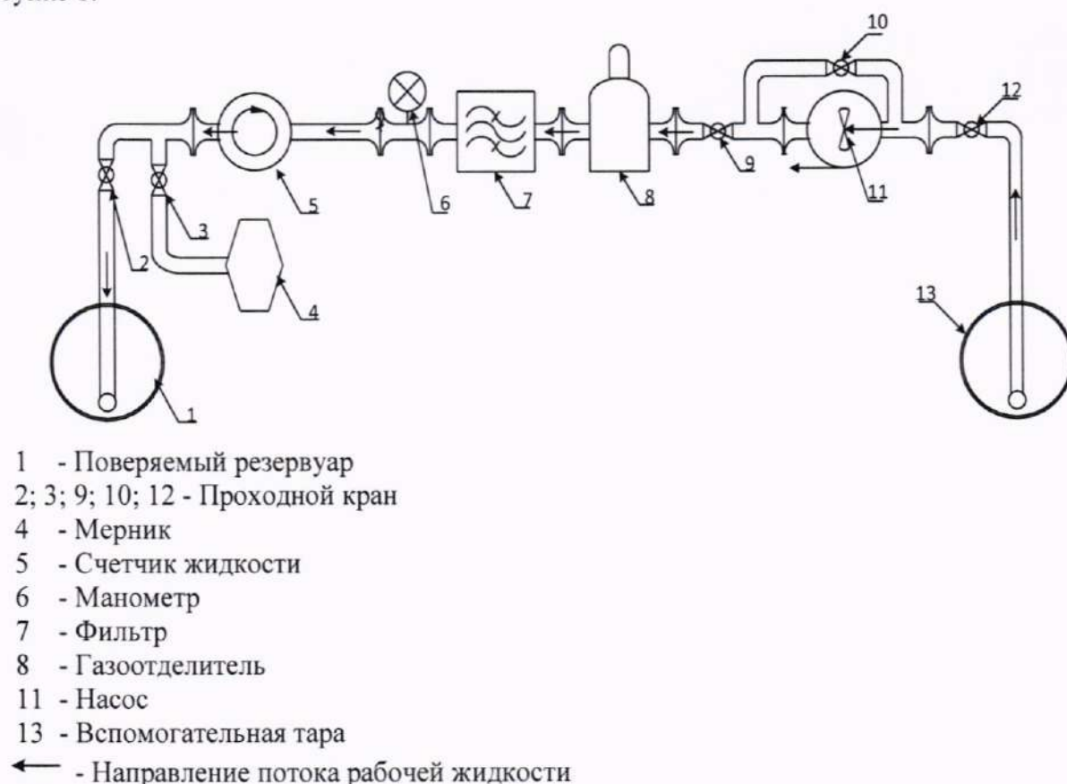
Рисунок 1 - Принципиальная схема установки поверочной передвижной КиПР
