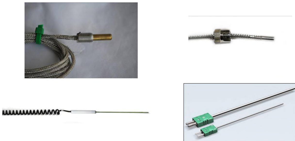
Рисунок 2 – Общий вид ДТП с кабельными выводами модификации XX4
