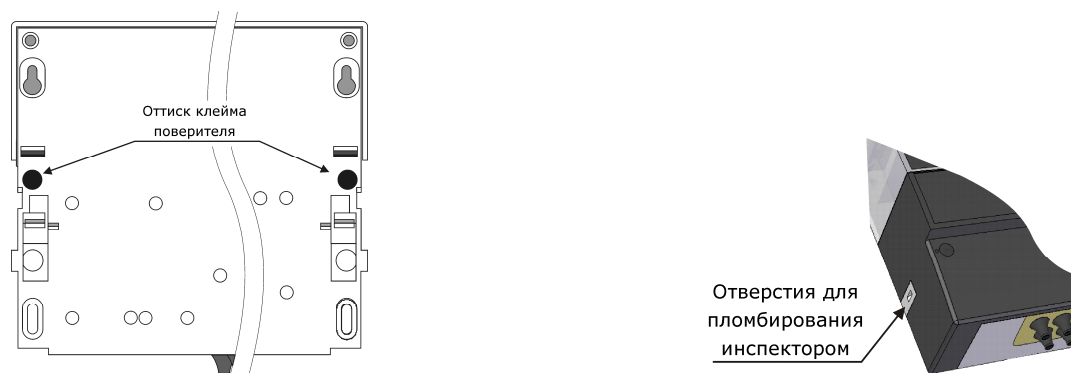
Рисунок 3 – Места пломбирования тепловычислителя
