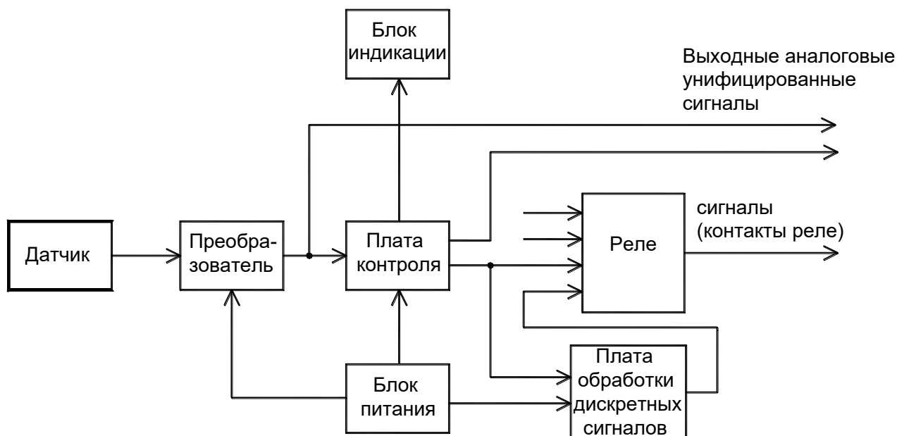
Рисунок 2 – Структурная схема
