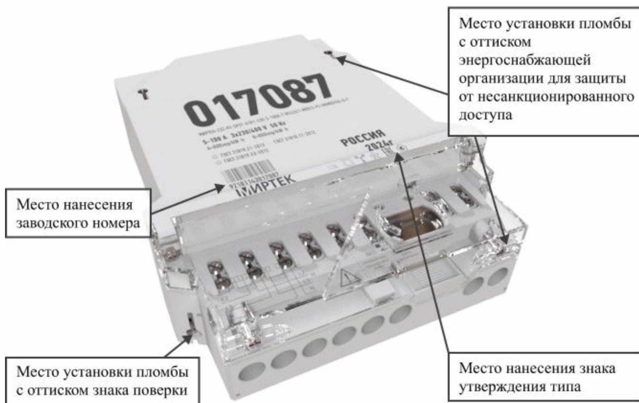
Рисунок 10 – Общий вид счетчика в корпусе типа SP31
