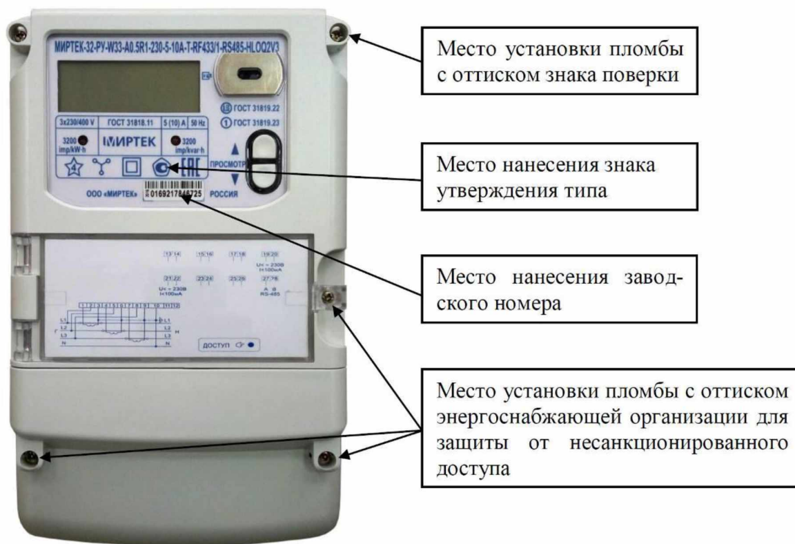
Рисунок 3 – Общий вид счетчика в корпусе типа W33
