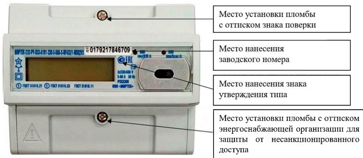
Рисунок 6 – Общий вид счетчика в корпусе типа D33
