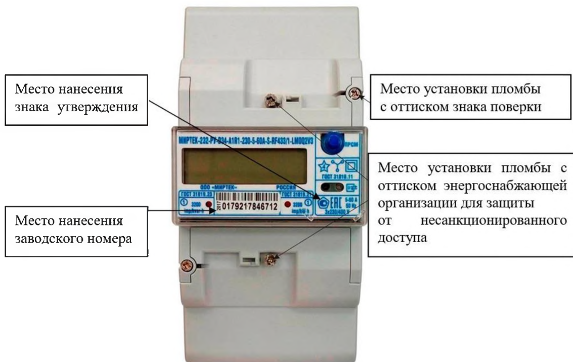
Рисунок 7 – Общий вид счетчика в корпусе типа D34
