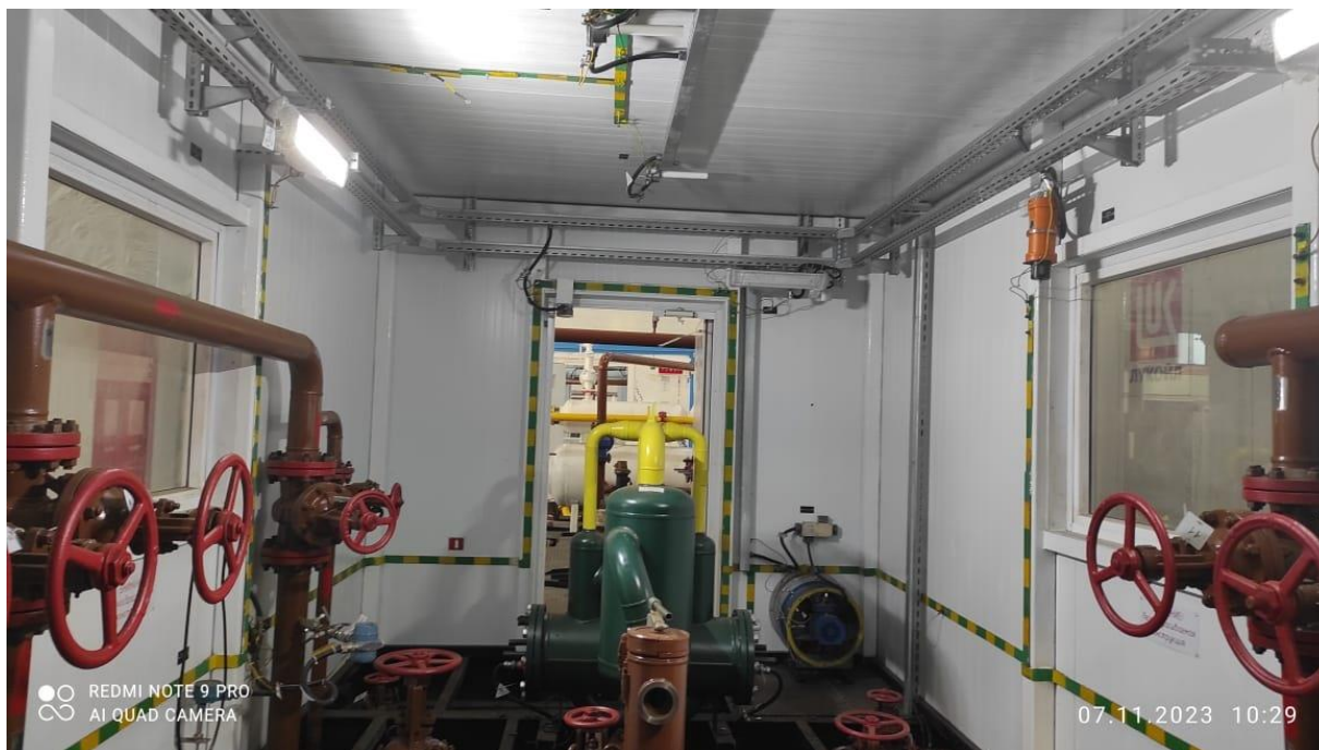
Рисунок 3 – Установка измерительная «МЕРА-ММ.ХХХ». Общий вид. Блок технологический бесепарационный
