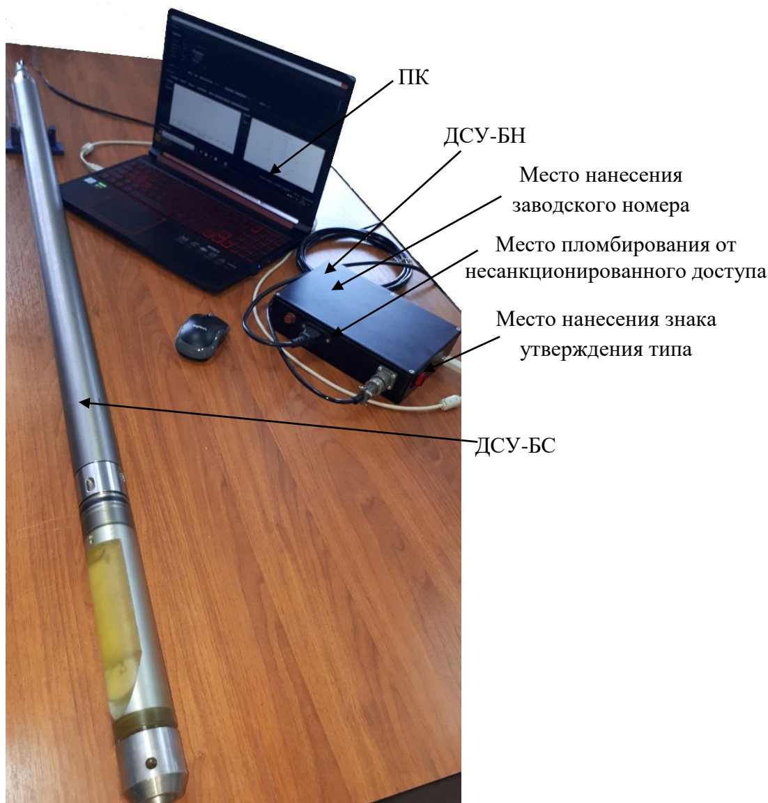
Рисунок 1 - Общий вид дальномеров
