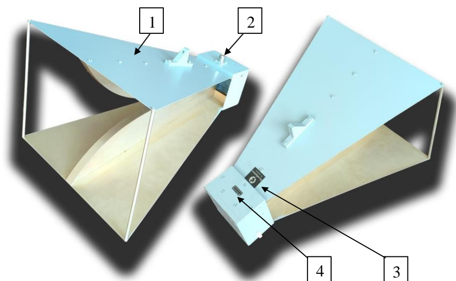
Рисунок 1 – Общий вид антенны П6-421 с указанием места пломбирования от несанкционированного доступа, места нанесения знака утверждения типа и заводского номера
