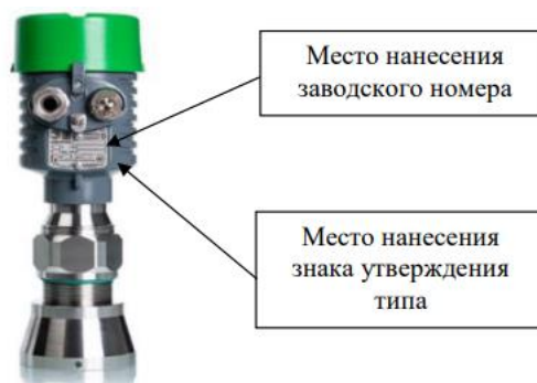
в) уровнемер с линзовой антенной
