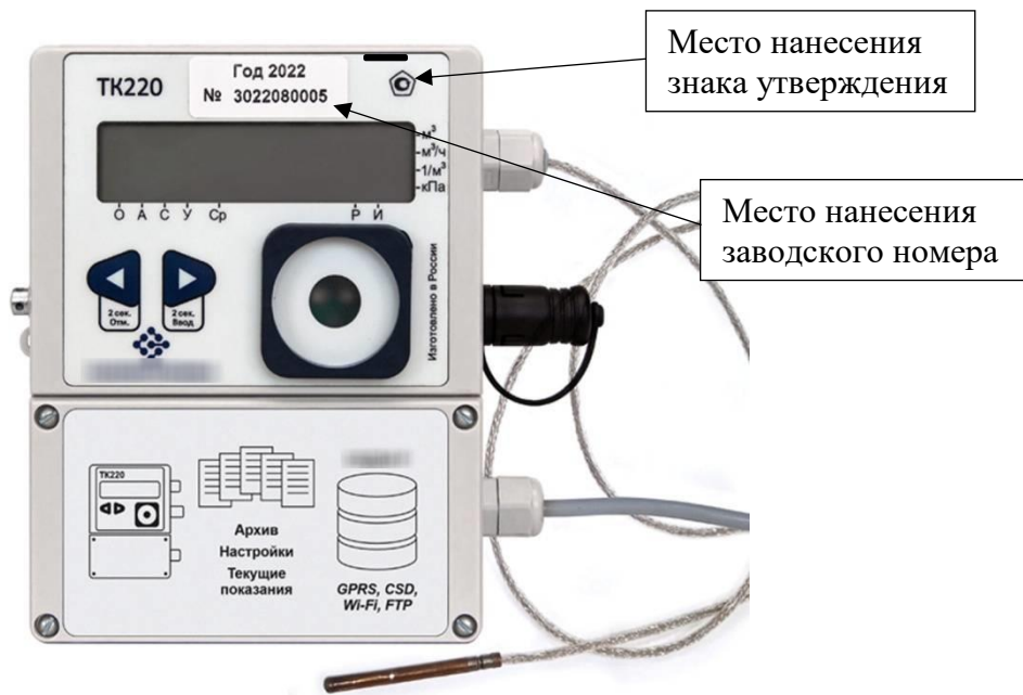
Рисунок 2 – Место нанесения заводского номера, знака утверждения типа
