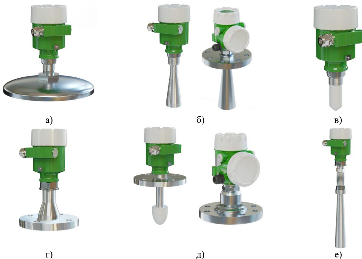
а) с параболической антенной; б) с конической антенной; в) с противокоррозионной антенной; г) с планарной антенной; д) с линзовой антенной; е) высокотемпературное исполнение Рисунок 2 – Общий вид уровнемеров
