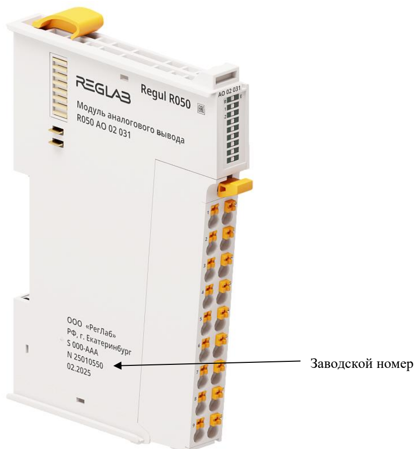
Рисунок 5 – Общий вид модулей контроллера REGUL R050
