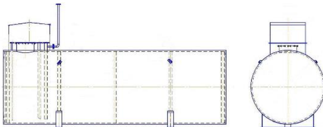
Рисунок 1 – Эскиз общего вида резервуаров РГС-25
