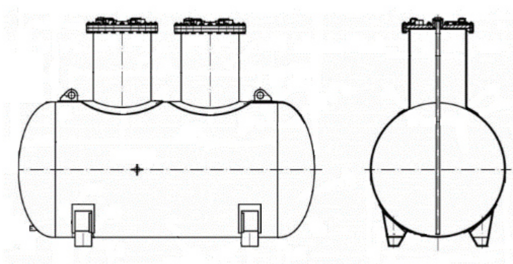
Рисунок 2 – Эскиз общего вида резервуаров РГС-50
