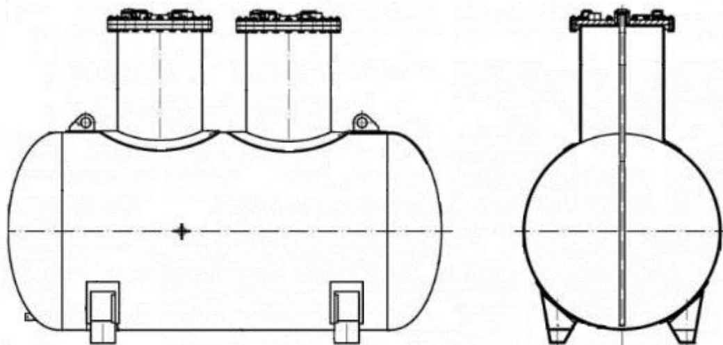
Рисунок 2 – Эскиз общего вида резервуара РГС-25 зав.№ 2
