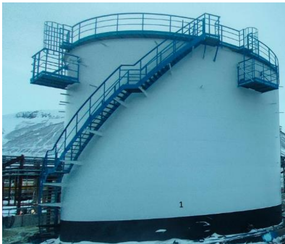
Рисунок 1 – Общий вид резервуара РВС-2000 № 1
