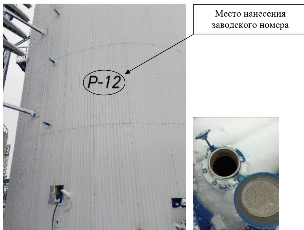
Р и с у н о к 4 – Общий вид резервуара с заводским номером P-12 и его замерного люка
