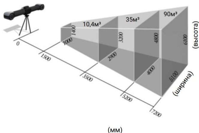
Рисунок 3 – Схема измерительных объёмов системы
