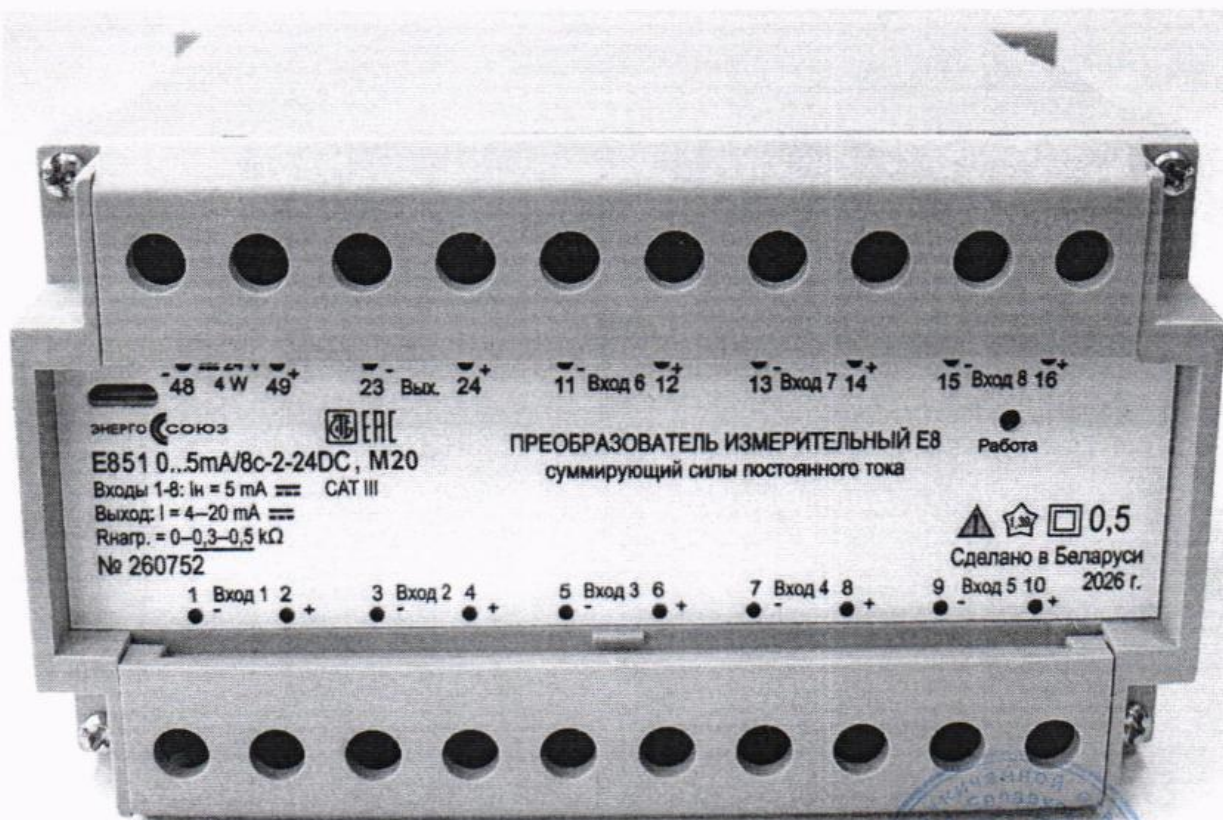
Рисунок 1.8 – Фотография модификации E851 в корпусе M20 (информация на табличке носит иллюстративный характер)
