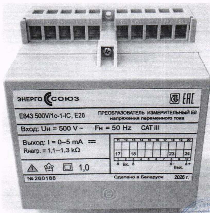
Рисунок 1.4 – Фотография модификации E843 в корпусе E20 (информация на табличке носит иллюстративный характер)
