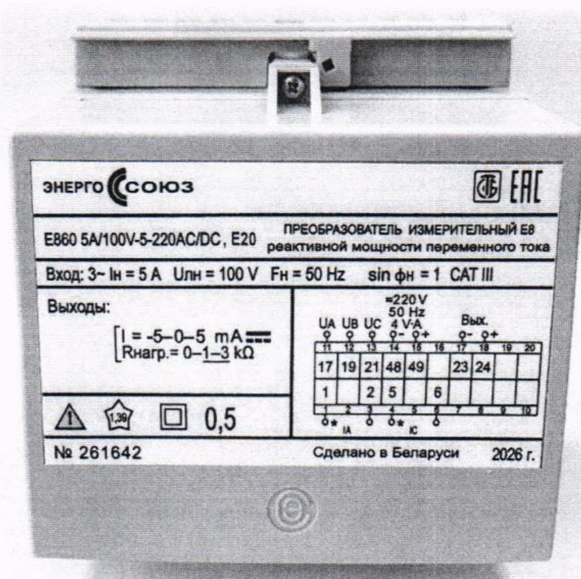
Рисунок 1.15 – Фотография модификации E860 в корпусе E20 (информация на табличке носит иллюстративный характер)
