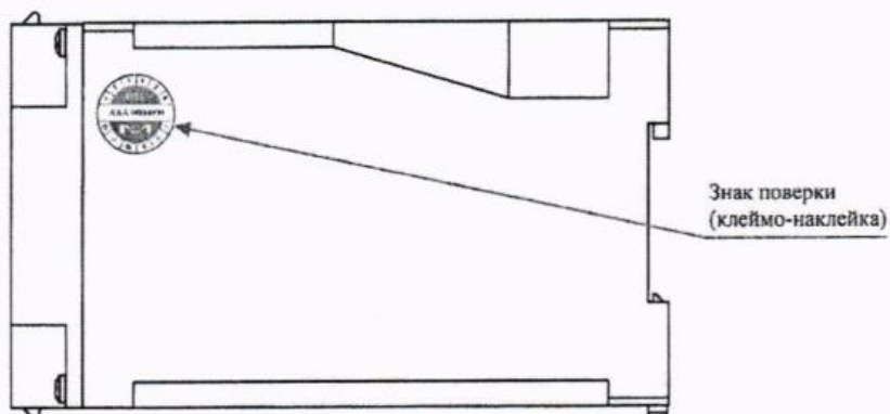
Рисунок 2.3 – Схема с указанием места для нанесения знака поверки на преобразователи в корпусах MB16
