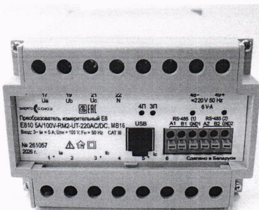
Рисунок 1.1 – Фотография модификации Е810 в корпусе МВ16 (информация на табличке носит иллюстративный характер)
