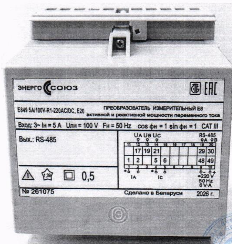
Рисунок 1.6 – Фотография модификации Е849 в корпусе Е20 (информация на табличке носит иллюстративный характер)
