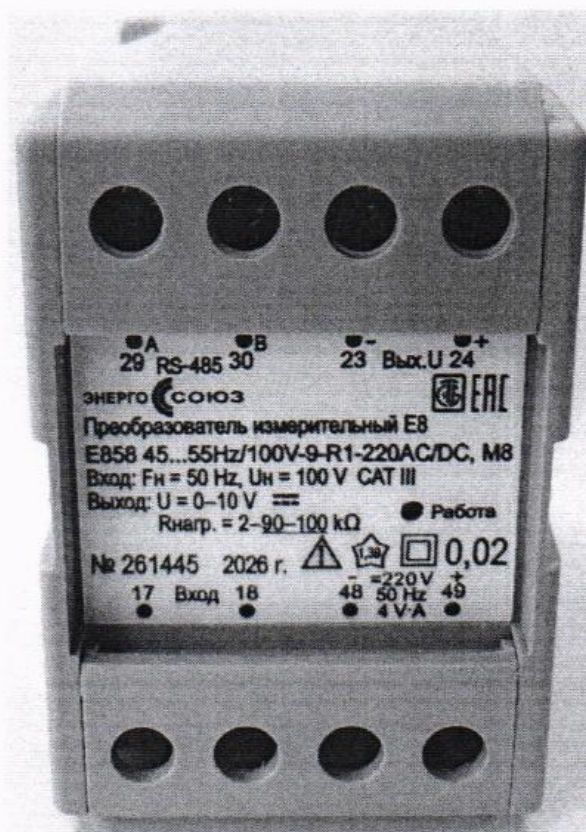
Рисунок 1.13 – Фотография модификации E858 в корпусе M8 (информация на табличке носит иллюстративный характер)
