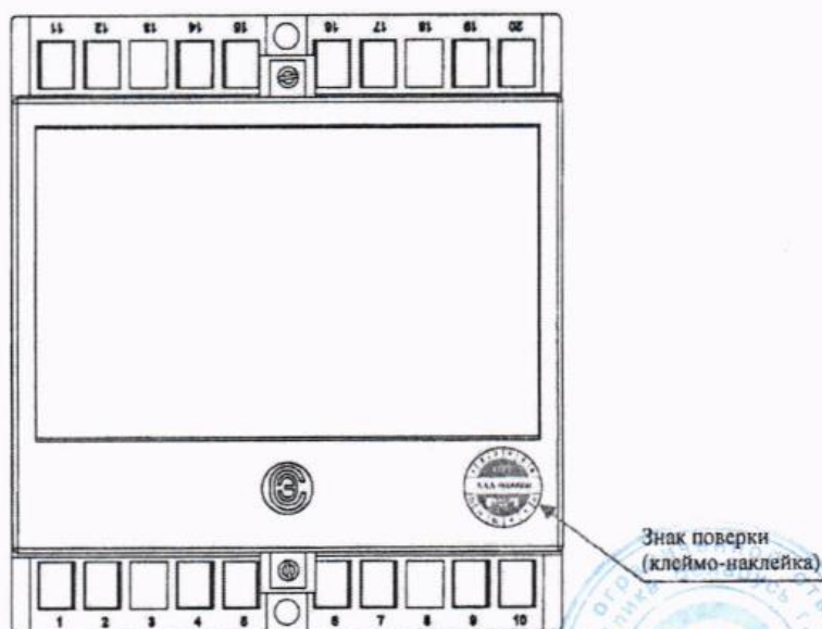
Рисунок 2.4 – Схема с указанием места для нанесения знака поверки на преобразователи в корпусах E20, EB20
