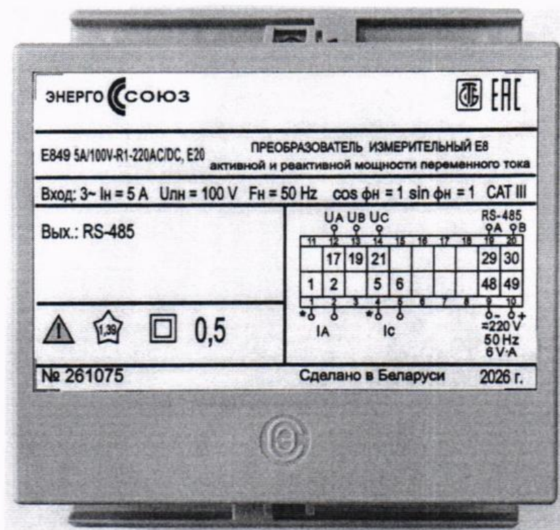
Рисунок 1.17 – Пример маркировки модификации Е849 (информация на табличке носит иллюстративный характер)
