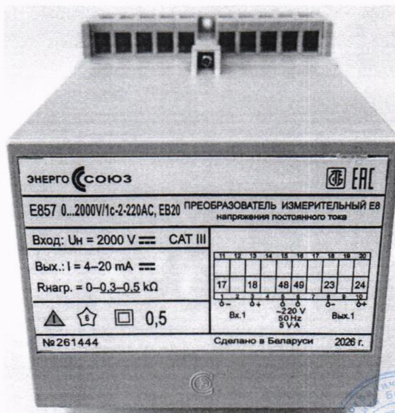
Рисунок 1.12 – Фотография модификации Е857 в корпусе EB20 (информация на табличке носит иллюстративный характер)
