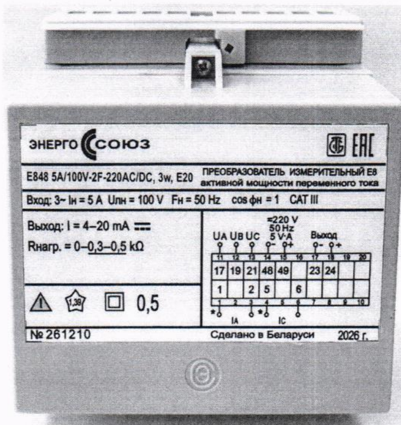
Рисунок 1.5 – Фотография модификации Е848 в корпусе Е20 (информация на табличке носит иллюстративный характер)
