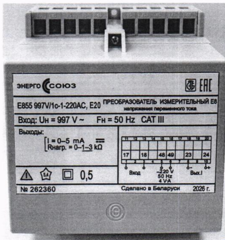
Рисунок 1.10 – Фотография модификации E855 в корпусе E20 (информация на табличке носит иллюстративный характер)
