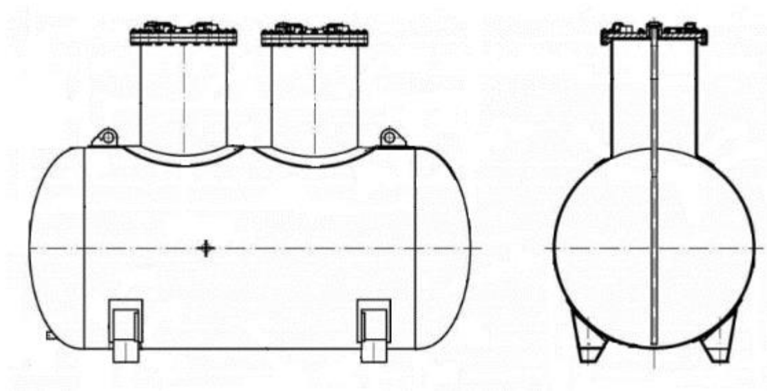
Рисунок 1 – Эскиз общего вида резервуаров РГС-15
