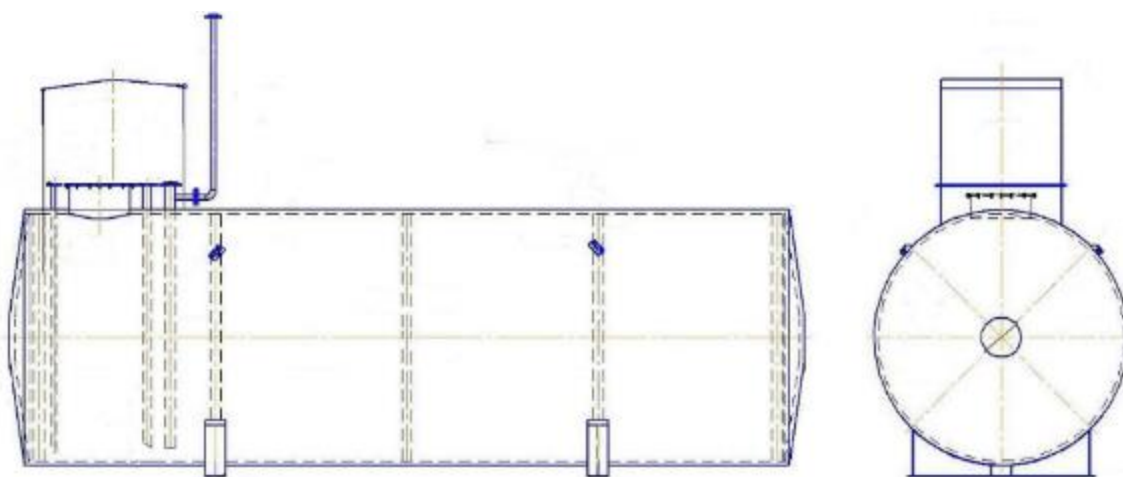
Рисунок 1 – Эскиз общего вида резервуаров РГС
