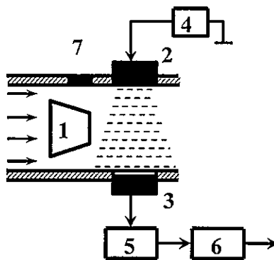
Рисунок 1.2 - Блок-схема преобразователя
