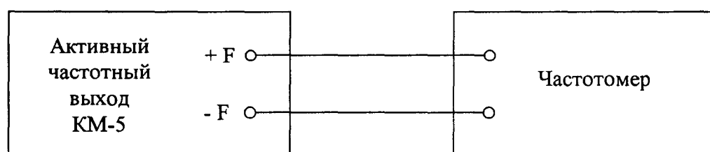
Рис. П1б. Электрическая схема подключения измерительных приборов при поверке частотного выхода КМ-5.
