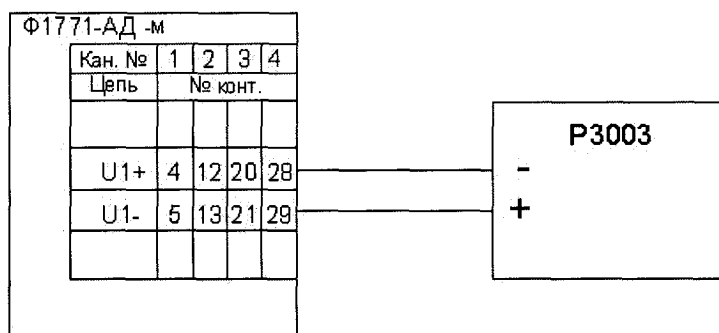
Рисунок 37 – Схема подключения входных каналов для U в диапазонах до \pm 2 В и сигналов ТП.
