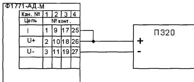
Рисунок 39 – Схема подключения входных каналов для постоянного тока
