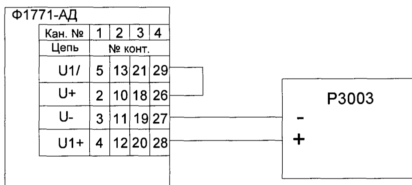
Рисунок 37 – Схема подключения входных каналов для U в диапазонах до \pm 2 В и сигналов ТП.
