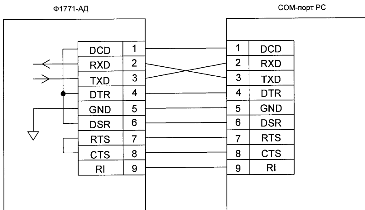
Рисунок 36- Схема соединения прибора Ф1771 с компьютером по интерфейсу RS232.
