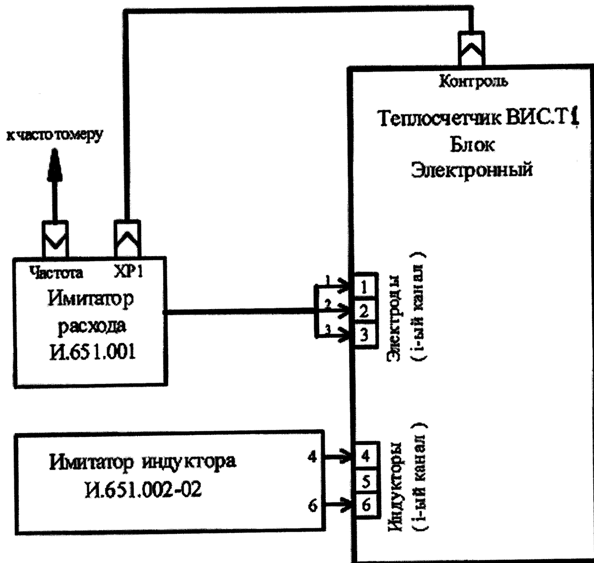
Схема подключения имитатора расхода
