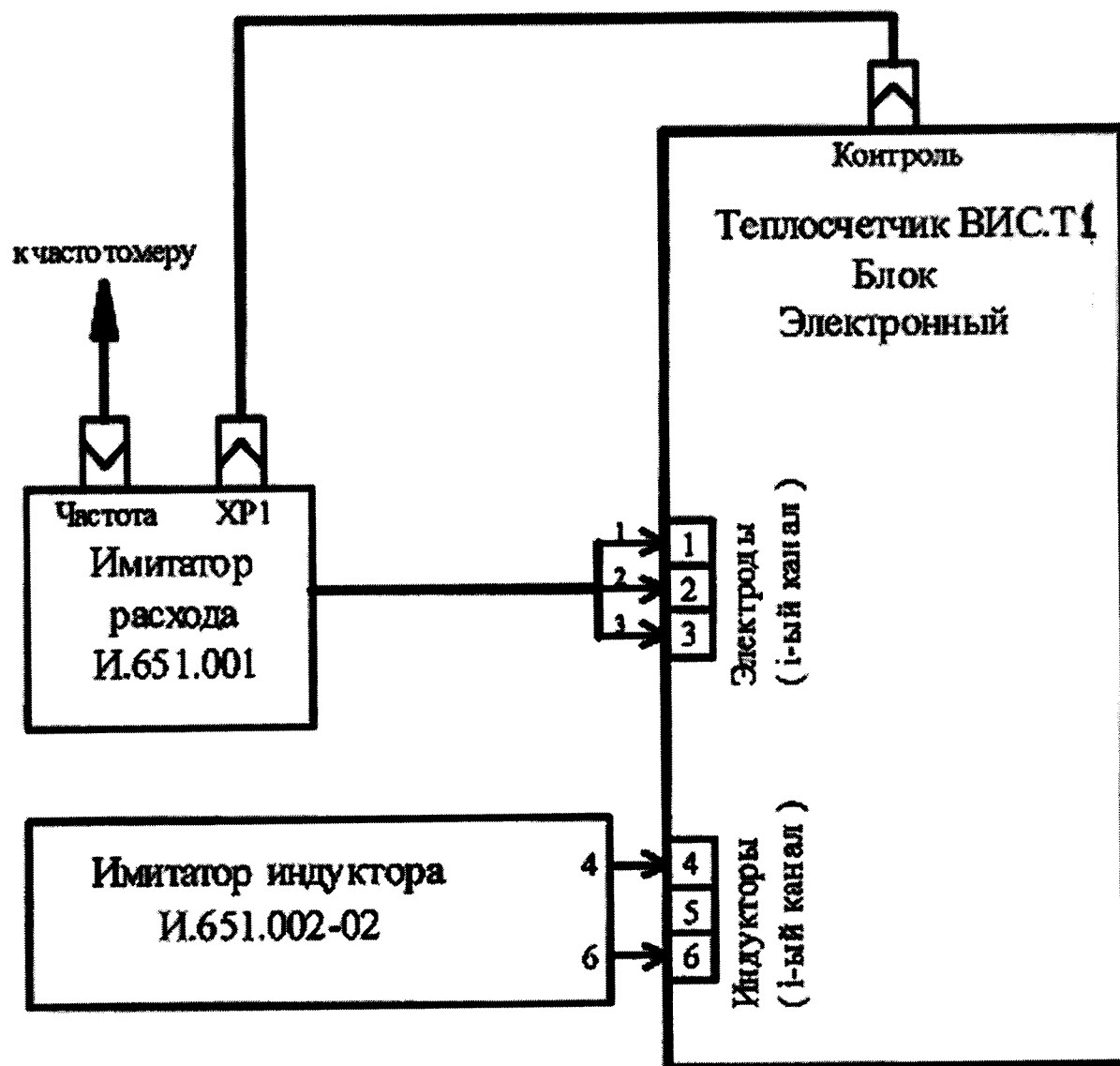
Схема подключения имитатора расхода
