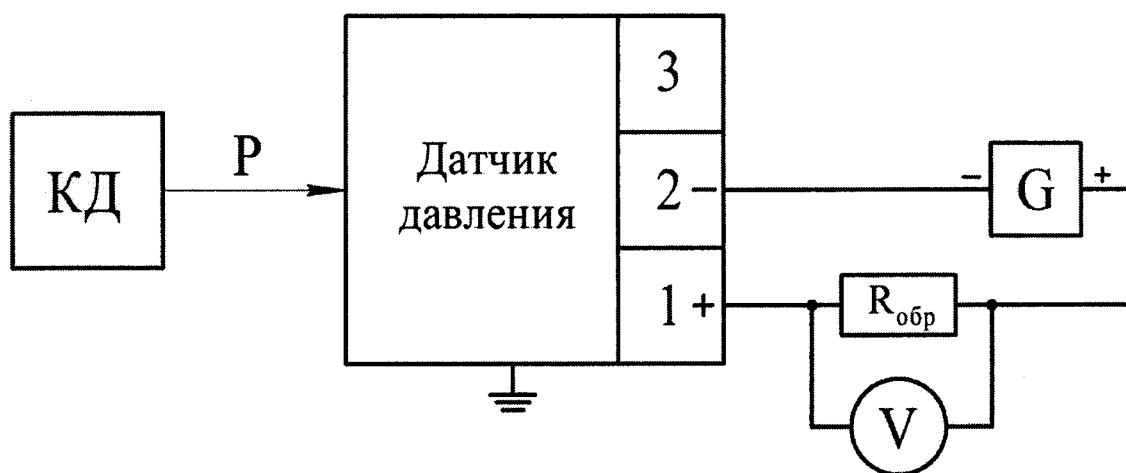
Рисунок А.1 – Схема включения датчиков давления с аналоговым выходным сигналом постоянного тока от 4 до 20 мА (от 20 до 4 мА) при измерении выходного сигнала непосредственно миллиамперметром
