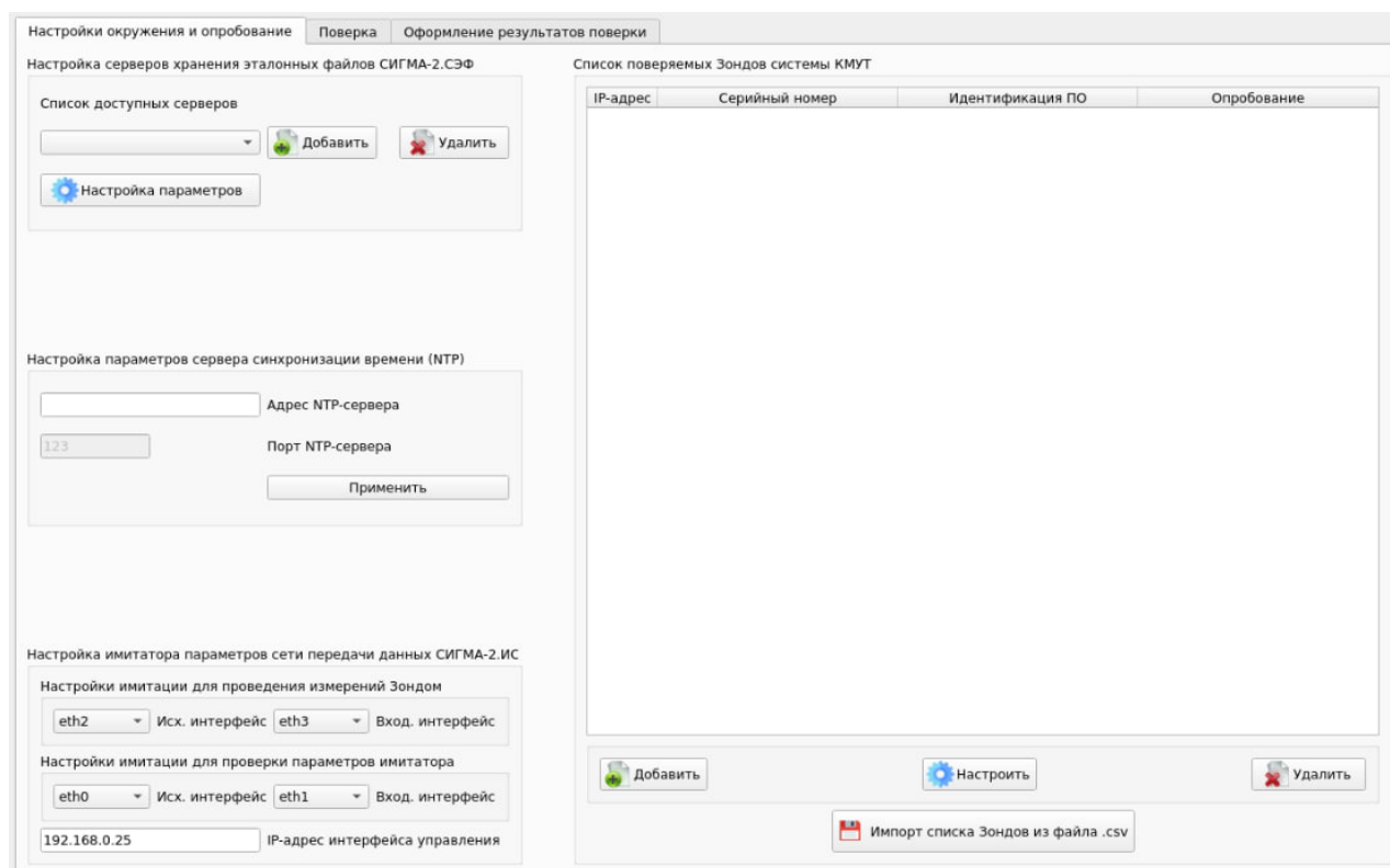
Рисунок 4 – Основное окно интерфейсного ПО СИГМА-КМУТ-Контроль
