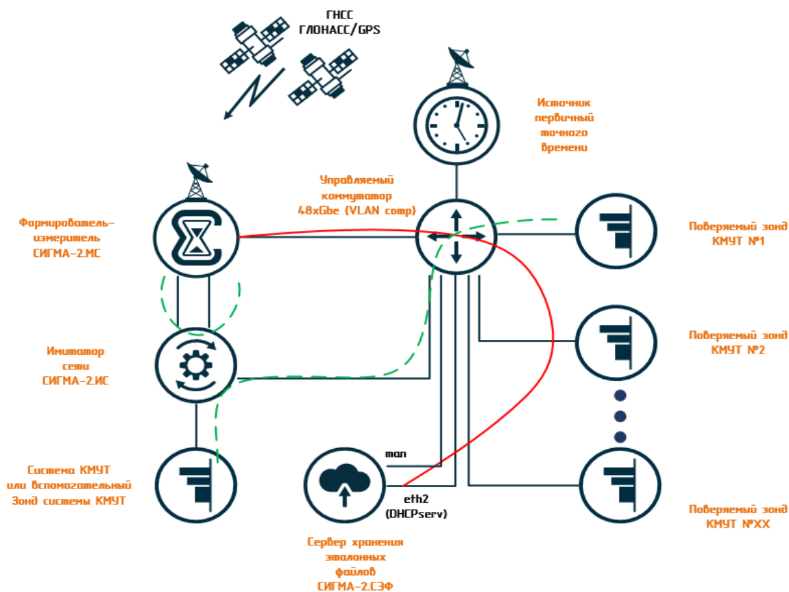
Рисунок 7 – Схема измерений при поверке Зонда КМУТ или сервера КМУТ
