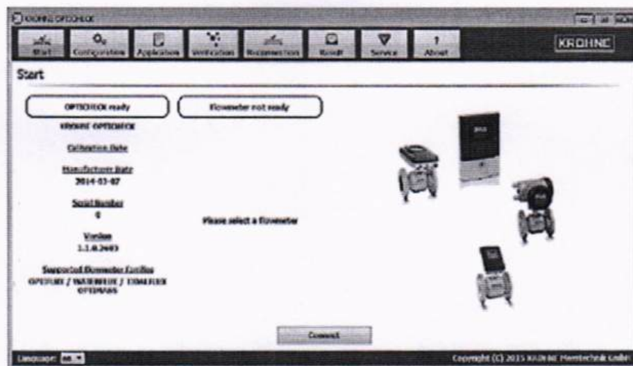
Рисунок 3 – Стартовое окно
