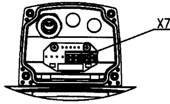
Клеммная коробка ПП. Вид сверху, крышка снята
