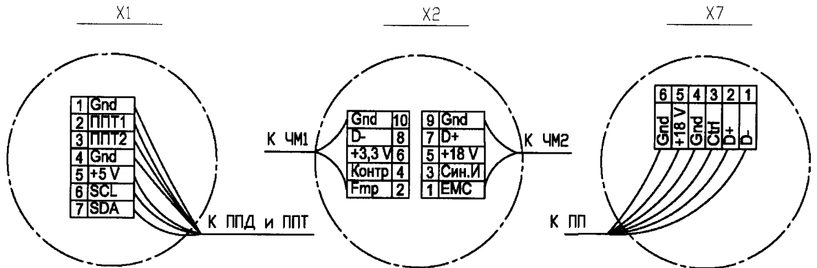
Рисунок 2 – Схемы подключения первичного преобразователя расходомера-счетчика
