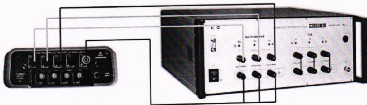
Рисунок 4 – Схема подключения приборов при определении погрешности измерения коэффициента n-ой гармонической составляющей напряжения, угла фазового сдвига между гармоническими составляющими напряжения
