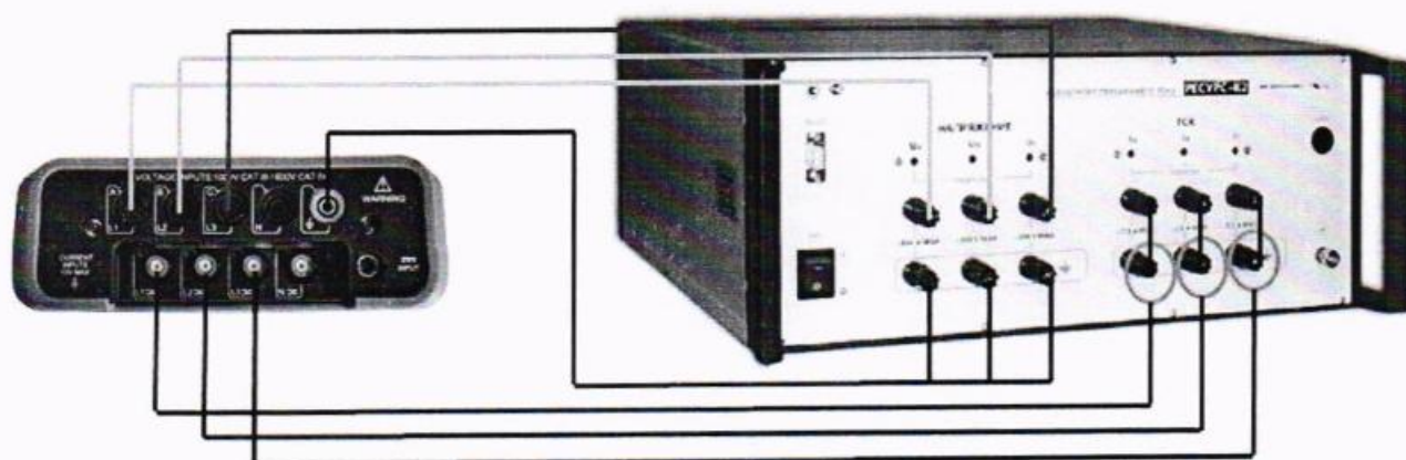
Рисунок 5 – Схема подключения приборов при определении погрешности измерения коэффициента n -ой гармонической составляющей тока, угла фазового сдвига между гармоническими составляющими тока
