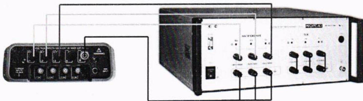
Рисунок 6 – Схема подключения приборов при определении погрешности измерения значений и длительности провалов и выбросов напряжения, коэффициента несимметрии напряжений, угла фазового сдвига между напряжениями основной частоты
