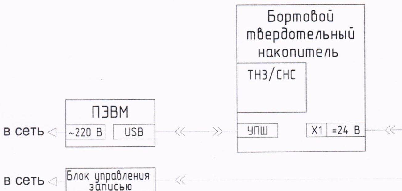
Рисунок 3 — Схема подключения модуля при проверке программного обеспечения
