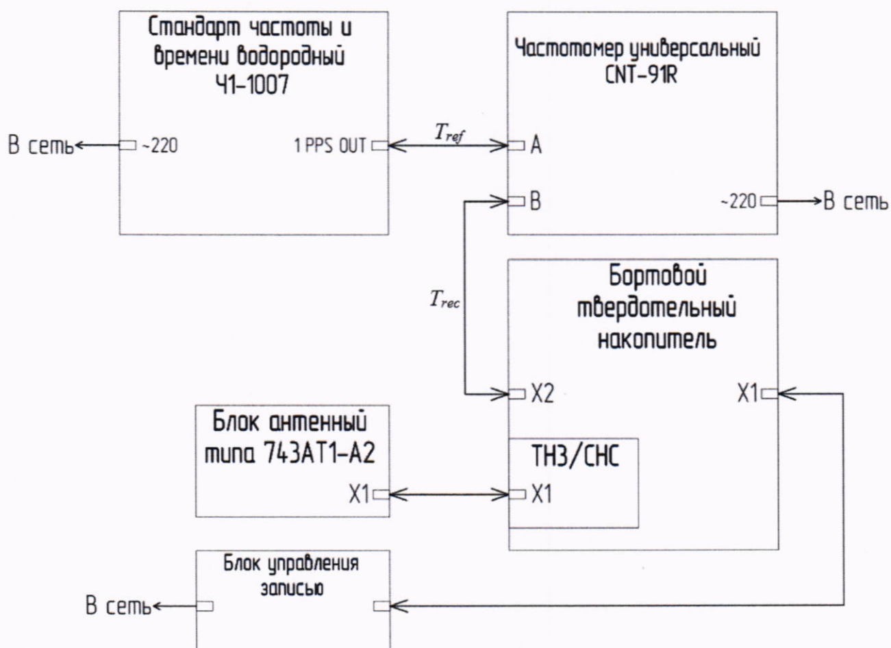
Рисунок 7 – Схема определения абсолютной погрешности синхронизации внутренней шкалы времени модуля с национальной шкалой координированного времени UTC(SU) при работе по сигналам ГЛОНАСС/GPS с применением блока антенного типа 743AT1-A2
