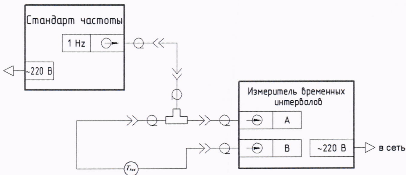
Рисунок А.1 – Схема измерения группового времени запаздывания в коаксиальном кабеле
