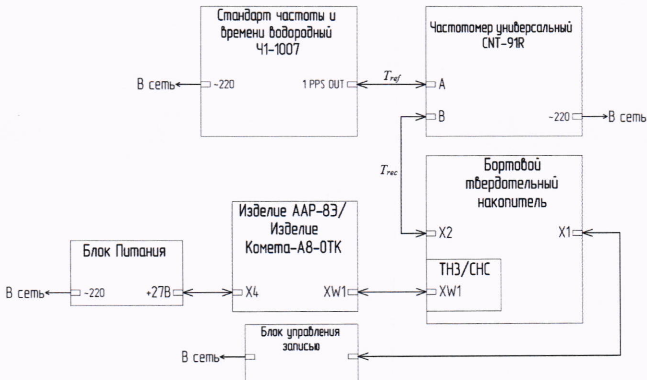
Рисунок 8 – Схема определения абсолютной погрешности синхронизации внутренней шкалы времени модуля с национальной шкалой координированного времени UTC(SU) при работе по сигналам ГЛОНАСС/GPS с применением изделия ААР-8Э или Комета-А8-ОТК
