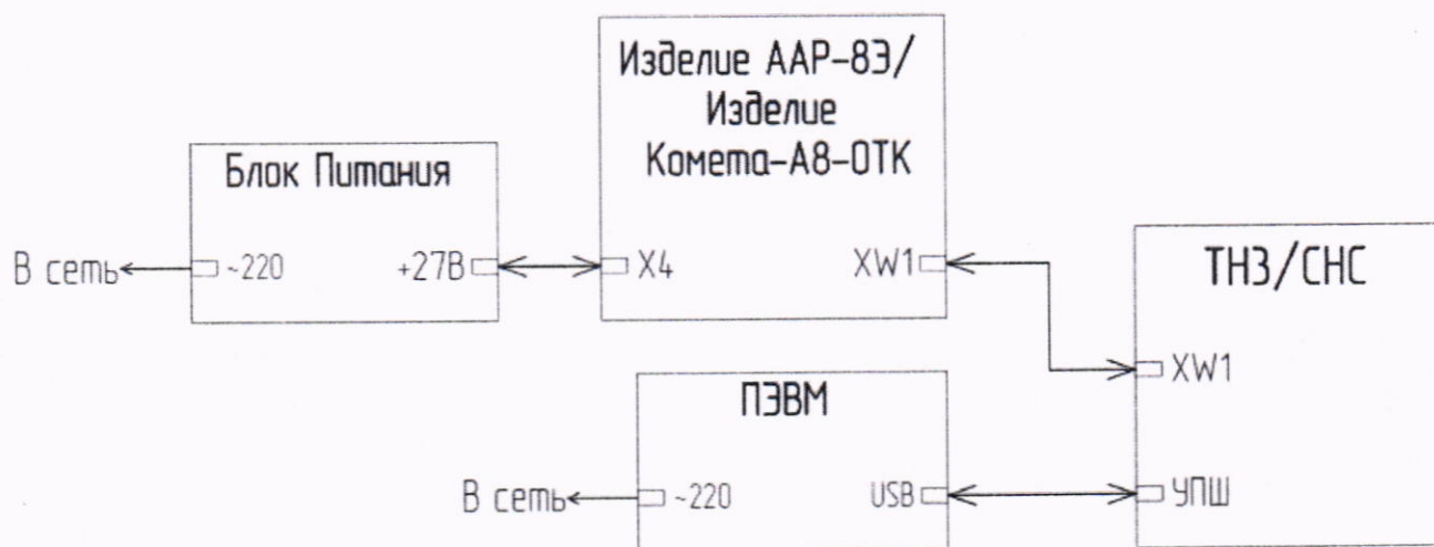
Рисунок 2 – Схема подключения модуля при проверке работоспособности с применением изделия ААР-8Э или Комета-А8-ОТК
