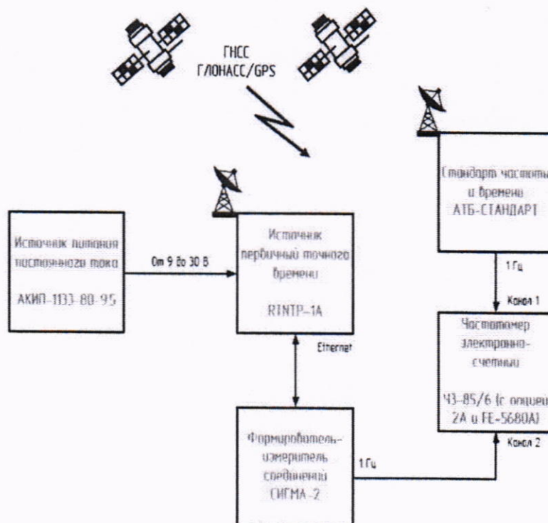
Рисунок 7. Схема измерений при определении абсолютной погрешности синхронизации формируемой шкалы времени с национальной шкалой времени UTC(SU) по протоколу NTP на интерфейсе Ethernet
