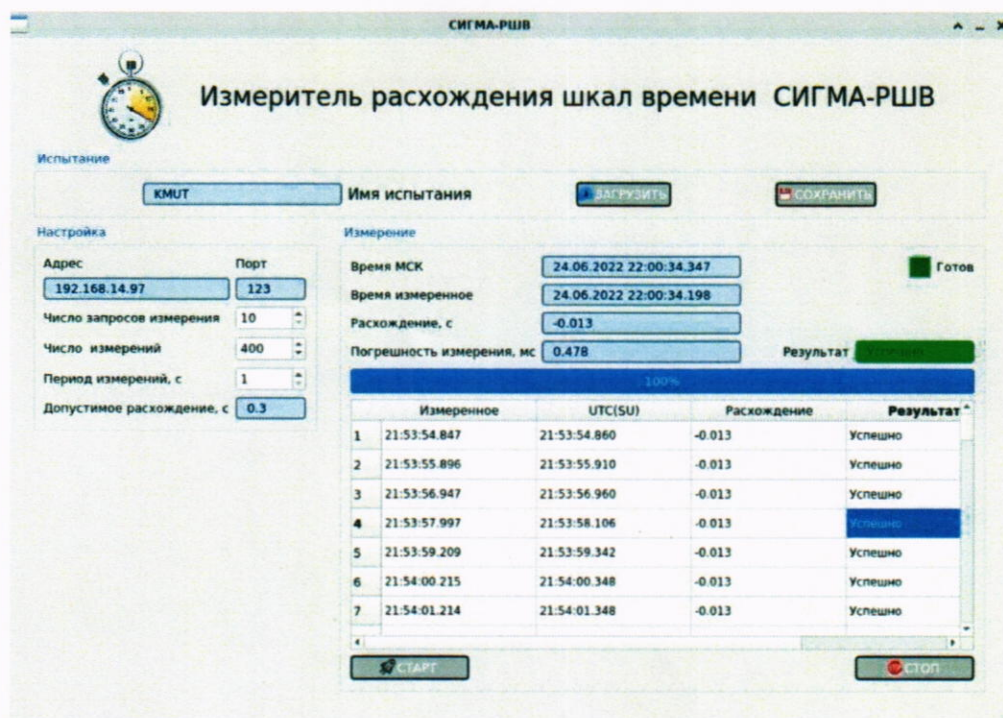
Рисунок 10. Индицирование результата испытаний подпрограммой СИГМА-РШВ
