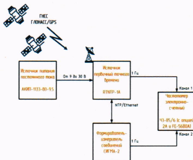
Рисунок 1 – Схема измерений для поверки
