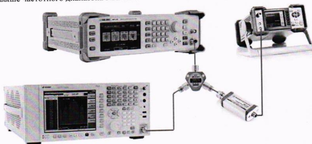
Рисунок 2 – Схема соединения приборов для определения погрешности установки выходного уровня генератора с использованием анализатора спектра N9030A
