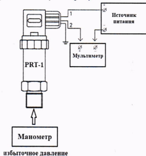
Рисунок 1 – Схема подключения
