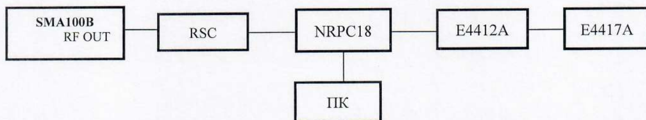
Рисунок 3 – Структурная схема соединения СИ для определения относительной погрешности измерений мощности для уровней мощности минус 70 дБ (1 мВт)
