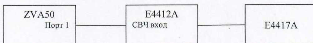
Рисунок 1 – Структурная схема определения КСВН входа
