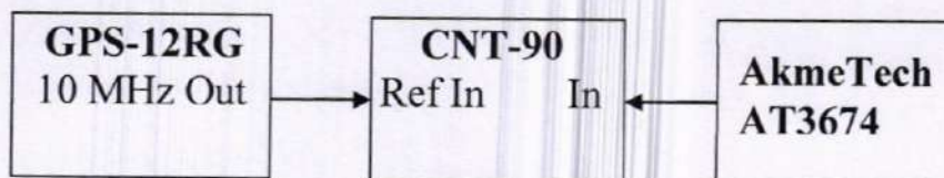
Рисунок 1 – Структурная схема определения относительной погрешности установки частоты опорного генератора
