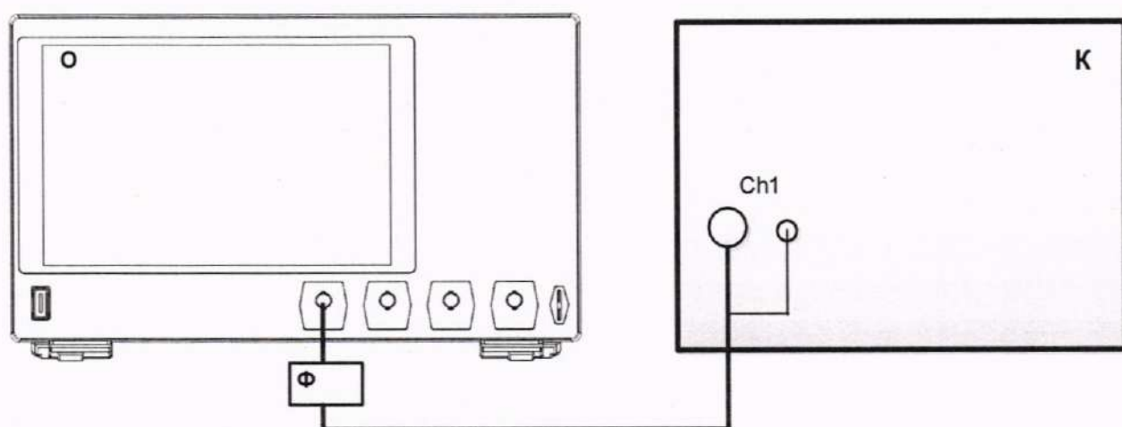
Рисунок 1- Схема подключения оборудования при определении значения входного сопротивления
