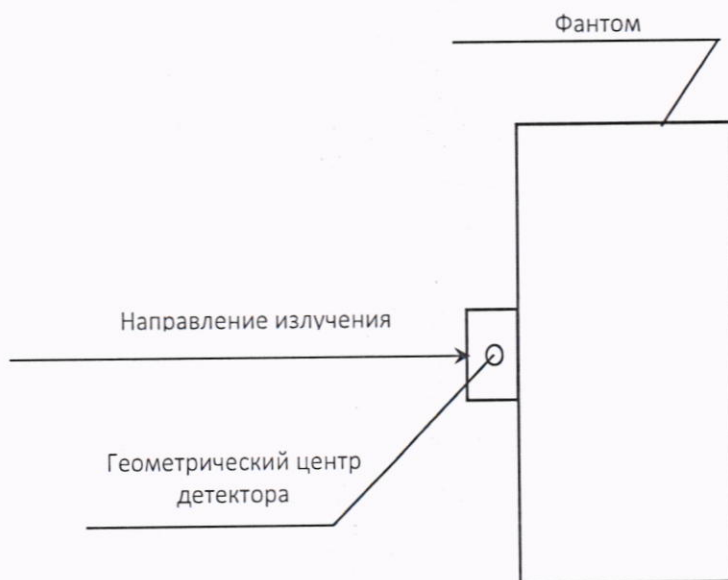
Рисунок 10.1 – Способ установки ДКГ-24А с фантомом на эталон
