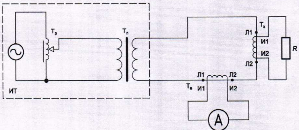
ИТ — регулируемый источник синусоидального тока; ~ — сеть (генератор); Т п — регулирующее устройство (автотрансформатор); Т п — понижающий силовой трансформатор; Т х — поверяемый трансформатор; Т в — вспомогательный трансформатор; R — резистор
