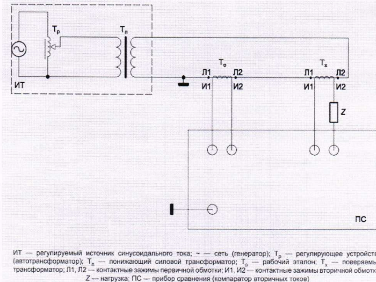
Рисунок 3 – Схема определения токовых и угловых погрешностей трансформаторов
